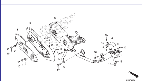
C-30 Escapamento
