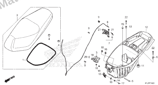
C-24 Assento • Compartimento de Bagagem
