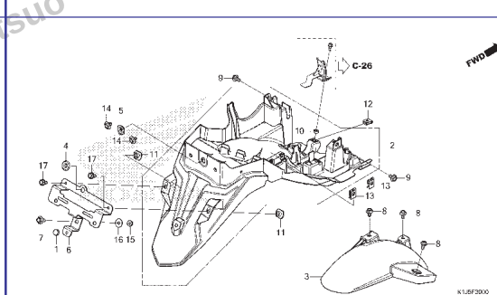
C-39 Para-lama Traseiro
