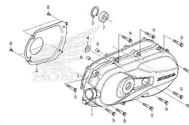
M-13 Tampa Lateral Esquerda
