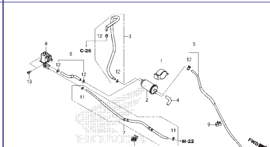
C-29 Câniseter
