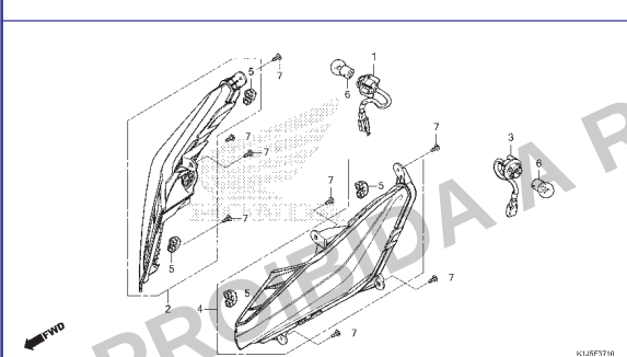
C-37.10 Sinalizador Dianteiro
