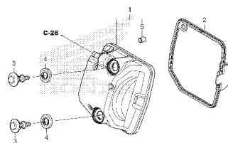
M-2 Tampa do Cabeçote
