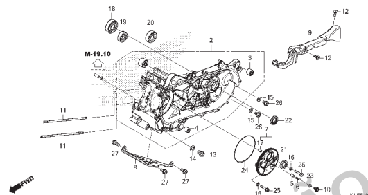
M-19.20 Carcaça do Motor Esquerda
