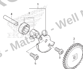
M-11 Bomba de Óleo
