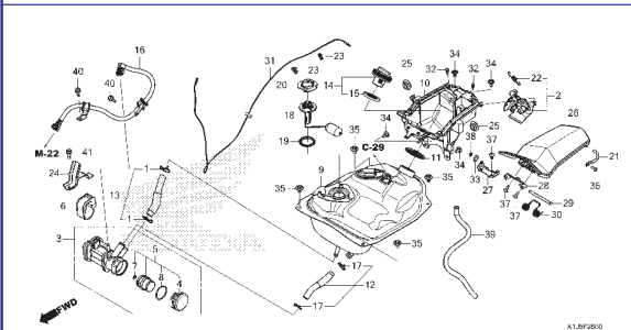
C-26 Tanque de Combustível • Bomba de Combustível
