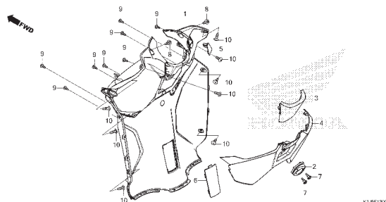
C-15 Tampa da Carcaça
