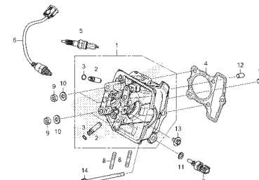
M-6 Cilindro
